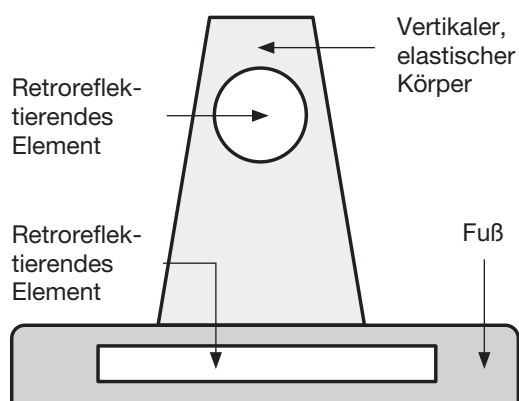
Bild 1: Schematische Darstellung eines Sichtzeichens
