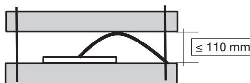
Bild 2: Belastungsversuch
