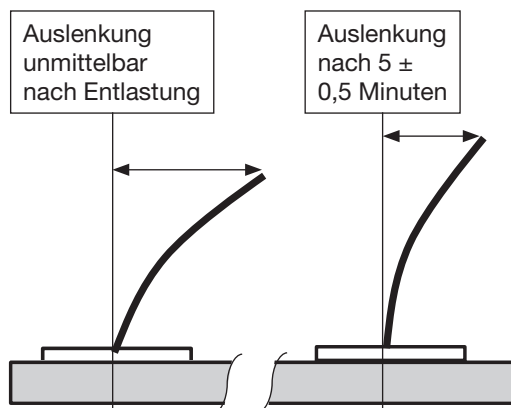
Bild 4: Auslenkung nach Belastung
